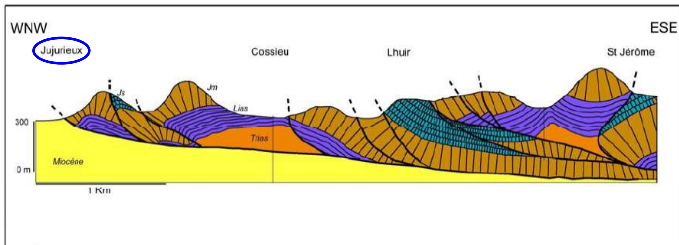
Coupe de Jujurieux à Saint Jérôme
